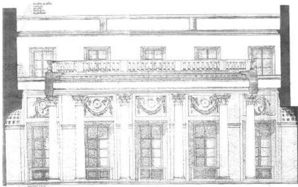
przekroj b-b 150
